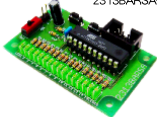
AVR2313/バーサライト基板キット 2313BARSA-KIT
