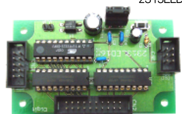
ATtiny2313+トランジスタアレイ基板キット 2313LED16
