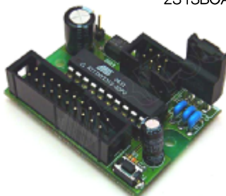
AVR ATtiny2313汎用基板キット 2313BOARD
